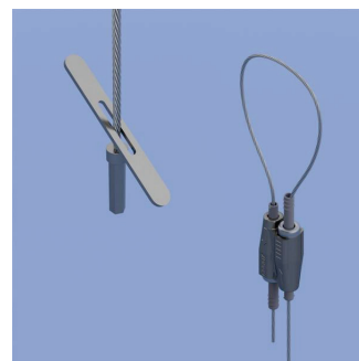
Speed Link SLK avec embout type bascule
